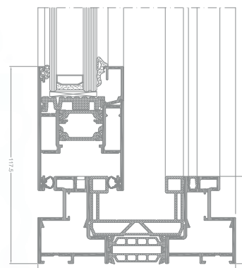
Vue en coupe d'une porte VG PLUS
