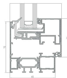
Coupe de fenêtre EF OC
