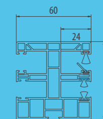
PVC PPDM 60/12 Rail de guidage utilisé dans les volets Opoterm avec moustiquaire intégrée. Vis employées – RD2
