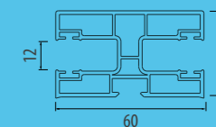
PG 02 Rail de guidage utilisé dans les volets à division.
