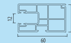
PG 08 Rail de guidage standard pour système CleverBox.
