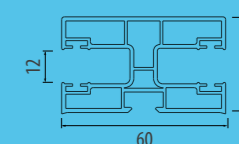
PG 02 Rail de guidage utilisé dans les volets à division.
