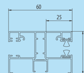
ALU PPDA 60/12 Équivalent en aluminium du rail de guidage standard pour système Opoterm. Vis employées – RD2
