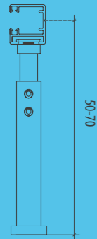
Fixation du rail de guidage de type TL
