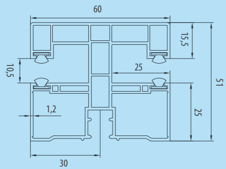
Rail de guidage de division
