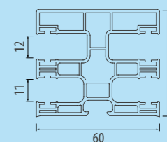
PG 09 Rail de guidage pour volet avec moustiquaire intégrée.
