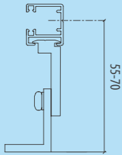
Fixation du rail de guidage de type N
