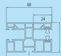
PVC PPD 60/12 Rail de guidage standard pour système Opoterm. Vis employées – RD2
